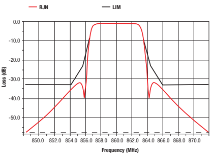
ATSC Stringent Mask
