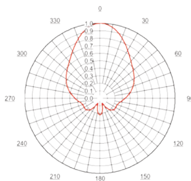
S380 3.97 (5.99 dB)
