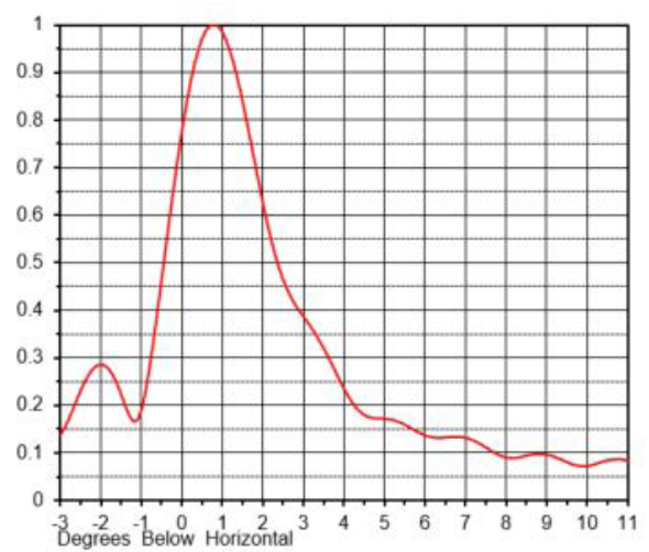
TFU-30EST-R
