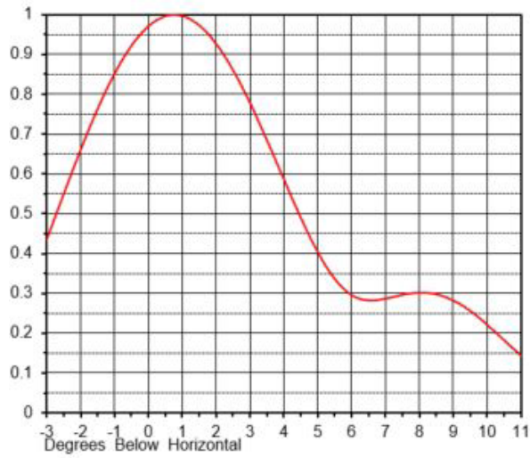
TFU-14EST-R
